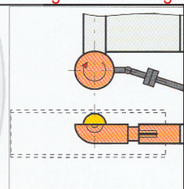
Longitudinal welding
